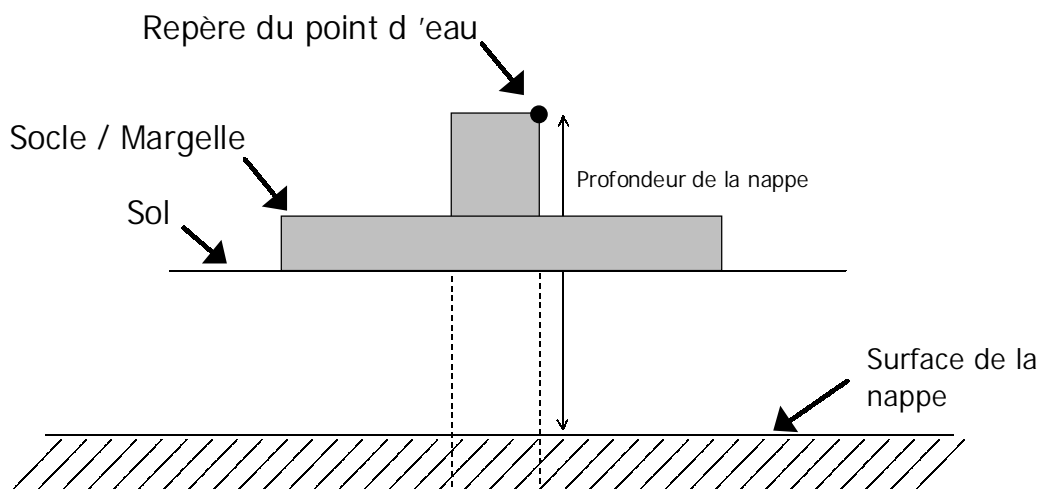
Figure 1 - Points remarquables du point d'eau
